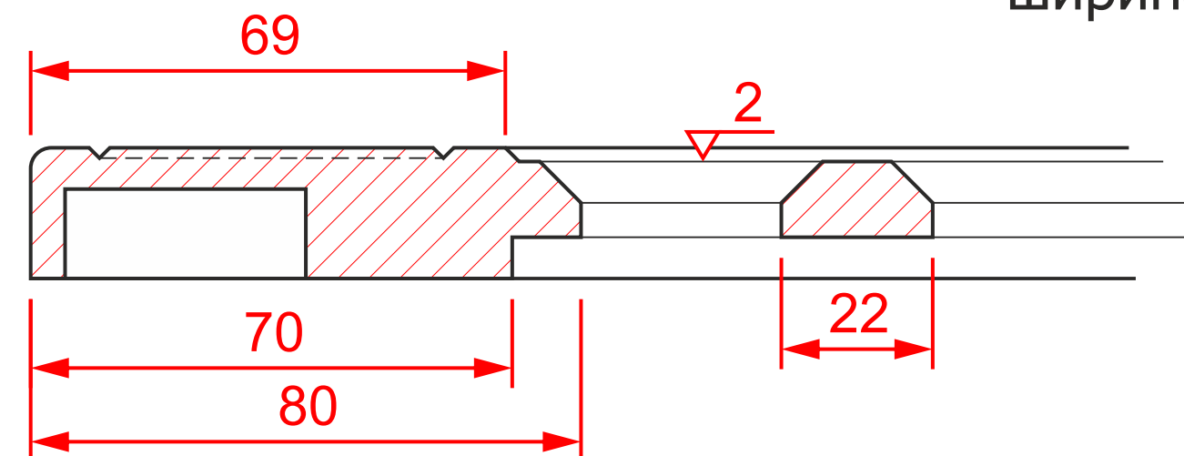
К-131 решетка2
