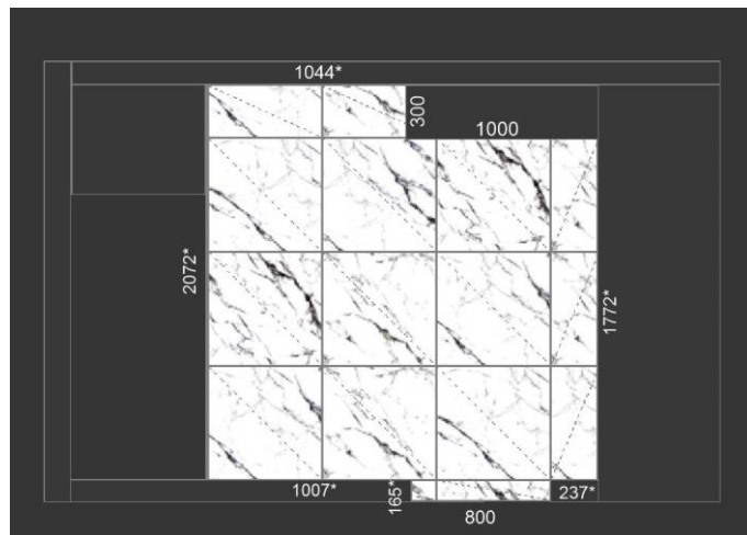
Раскладка плитки ванная
