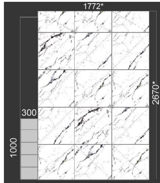
Раскладка плитки ванная
