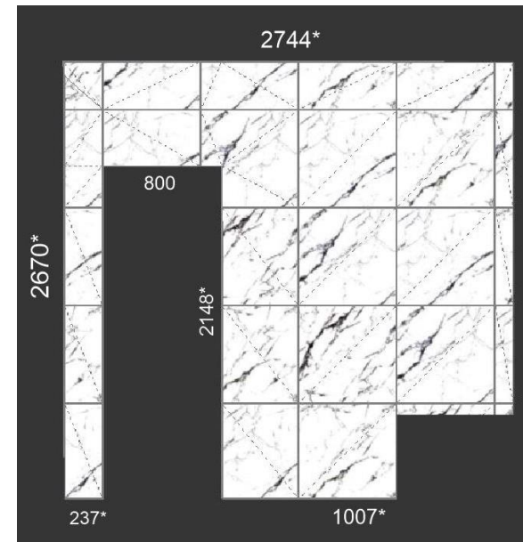
Раскладка плитки ванная
