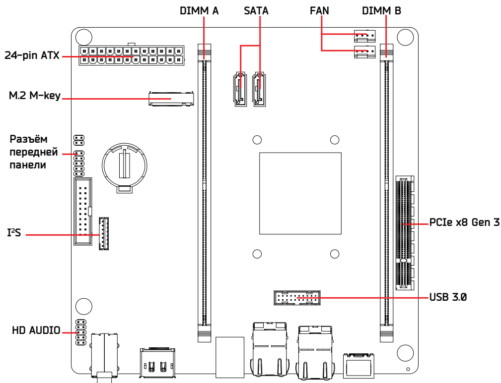
Рисунок 2 Расположение компонентов для исполнения ET101-MB-12
