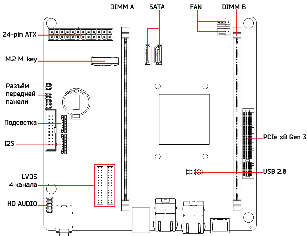
Рисунок 1 Расположение компонентов для исполнения ET101-MB-11
