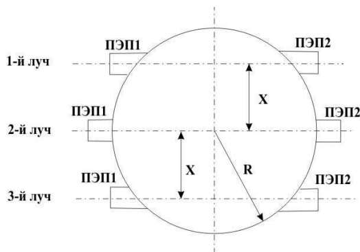
Рисунок 12 – Положение пар ПЭП для трехлучевых расходомеров
