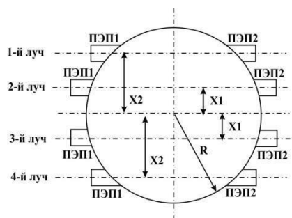
Рисунок 13 – Положение пар ПЭП для четырехлучевых расходомеров
