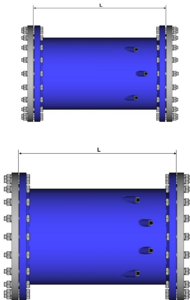
Рисунок 2 – Габаритные размеры и массы УПР
