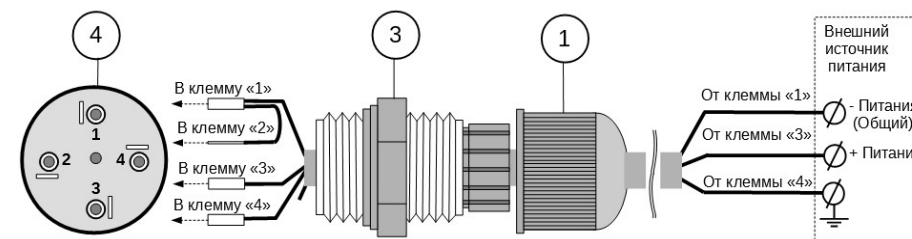
Рисунок 8 – Подключение внешнего кабеля к клеммам разъема
