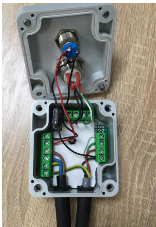
Рис. 3 - Внутренности коммутационной коробки № 1
