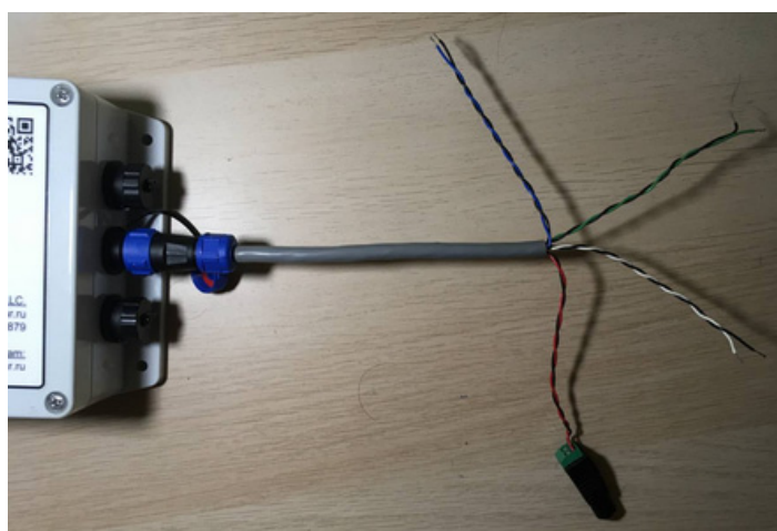
Рис. 9 - Кабель для разъема № 2 к трекеру из комплекта поставки
