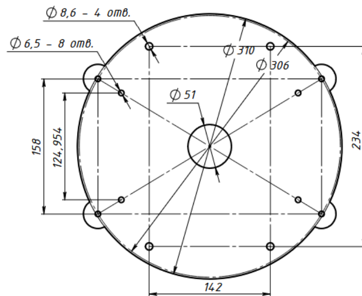
Рис. 2 Вид крепления КГ-02 сверху
