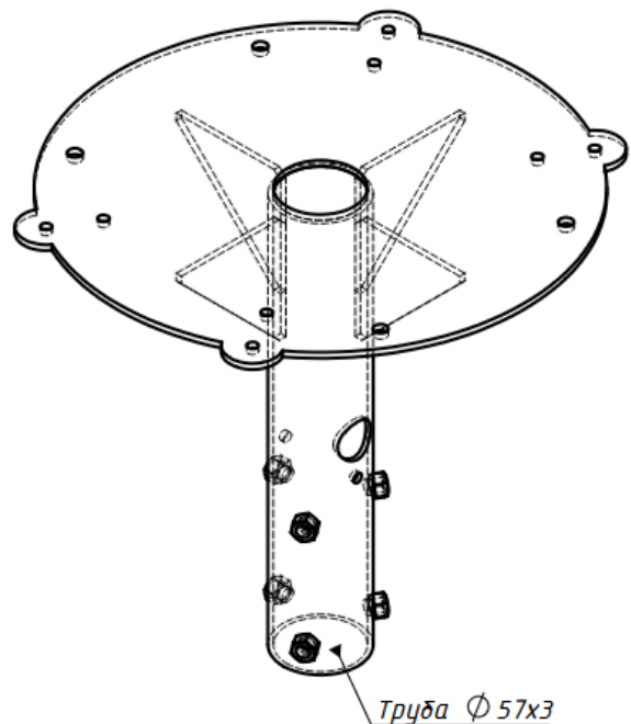
Рис. 1 – Внешний вид крепления КГ-02
