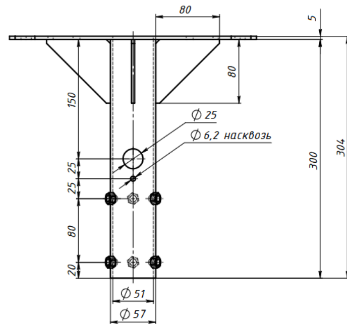
Рис. 2 Вид крепления КГ-02 сбоку
